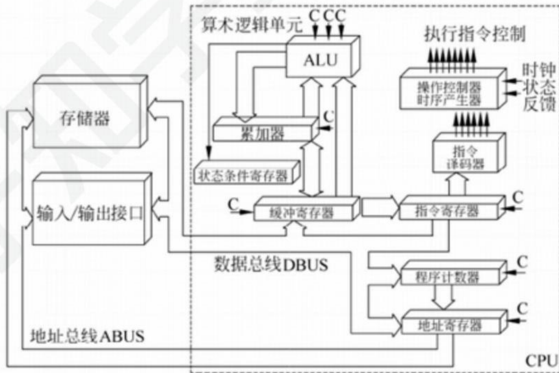
CPU 基本组成结构示意图
